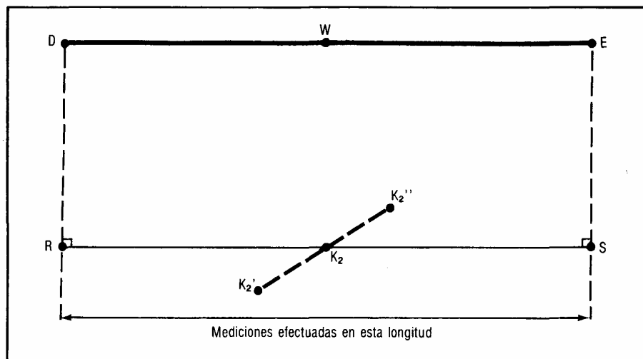
Figura 2-5. Perfil típico de sobrevuelo
